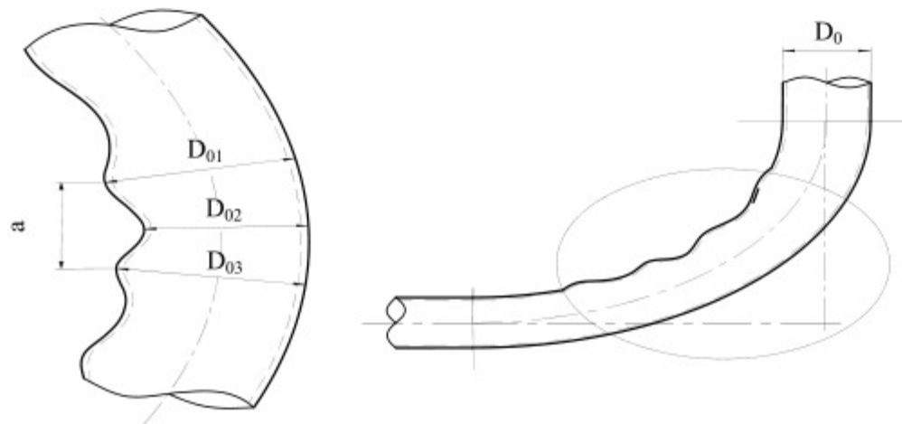
图 5.3.7-1 弯管的褶皱和波浪间距
