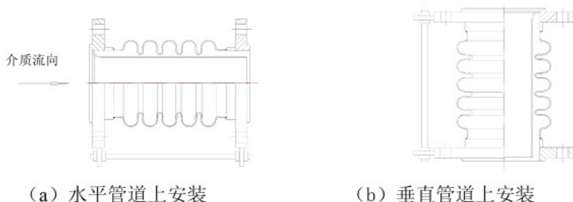
图 7.11.3 波纹管膨胀节在管道上的安装位置
