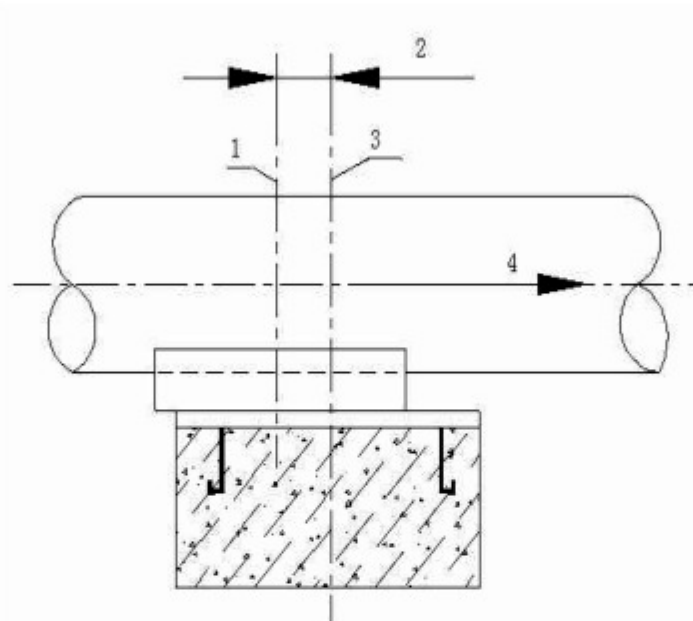
图 7.12.5 滑动支架安装位置
