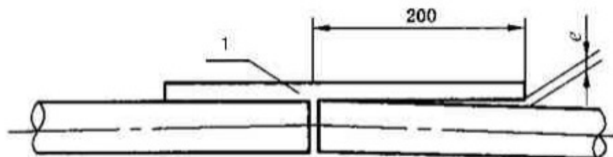
图 7.3.10 管道对口平直度
