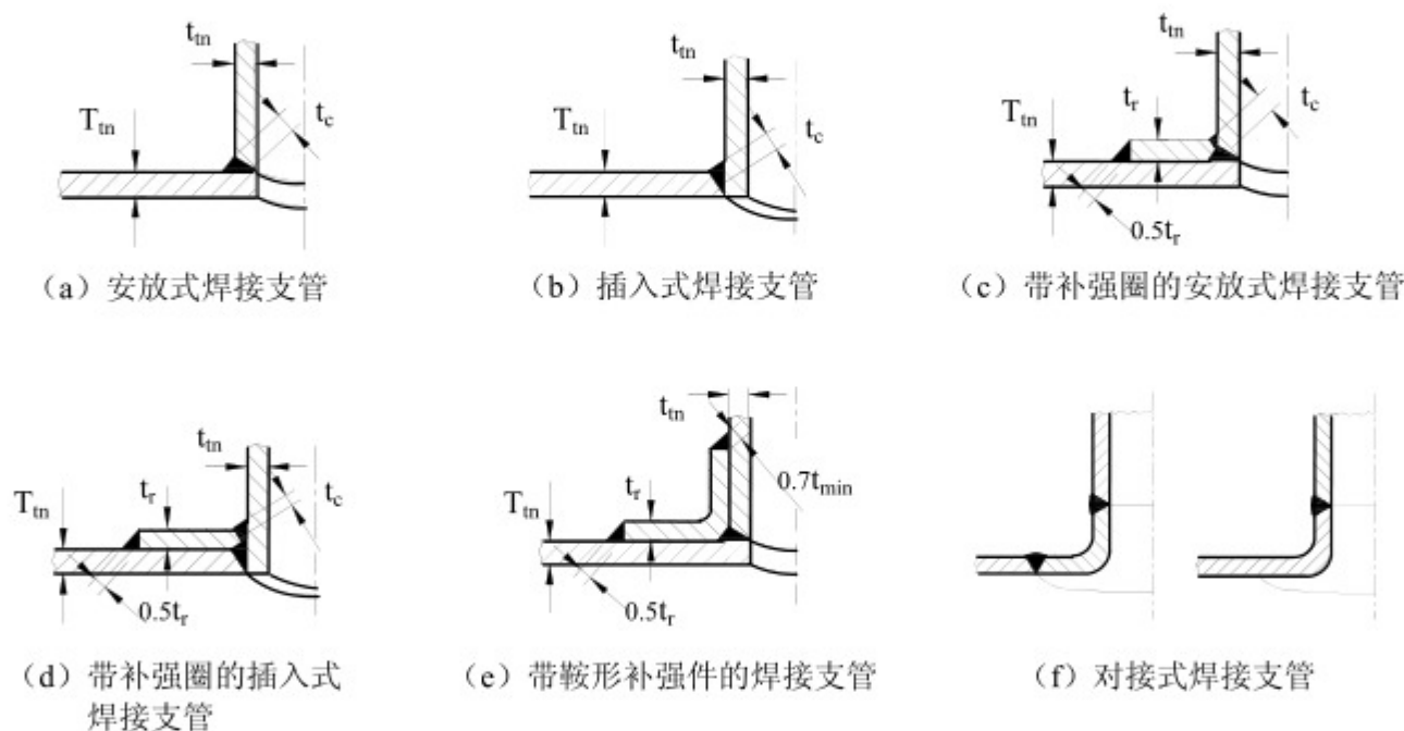
图 6.0.8 支管连接的焊缝形式
