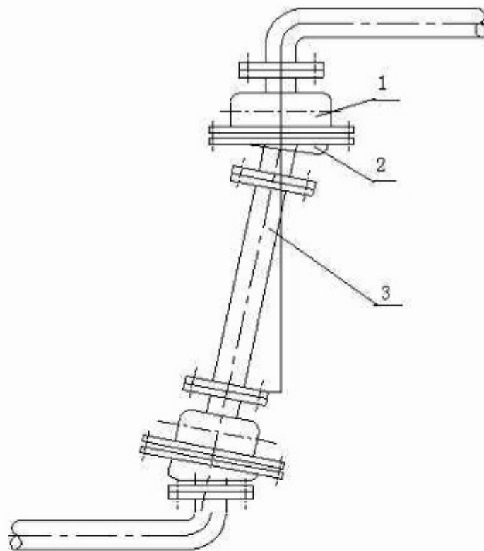
图 7.11.5—1 球形补偿器与球心距管段的组合
