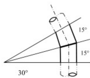
(d) 30° 斜接弯头
