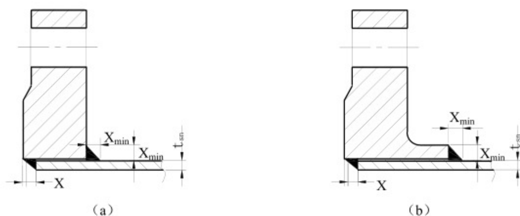
图 6.0.7-1 平焊法兰与管子的连接
