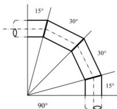
(a) 90° 斜接弯头
