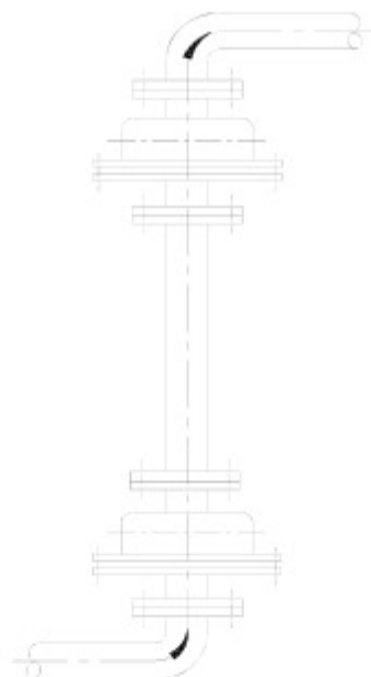
图 7.11.5—3 球形补偿器的安装方向
