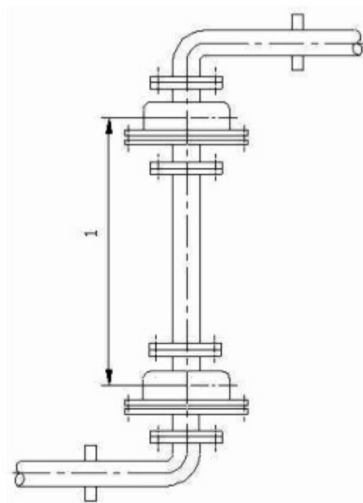
图 7.11.5—2 球形补偿器球心距的安装长度
