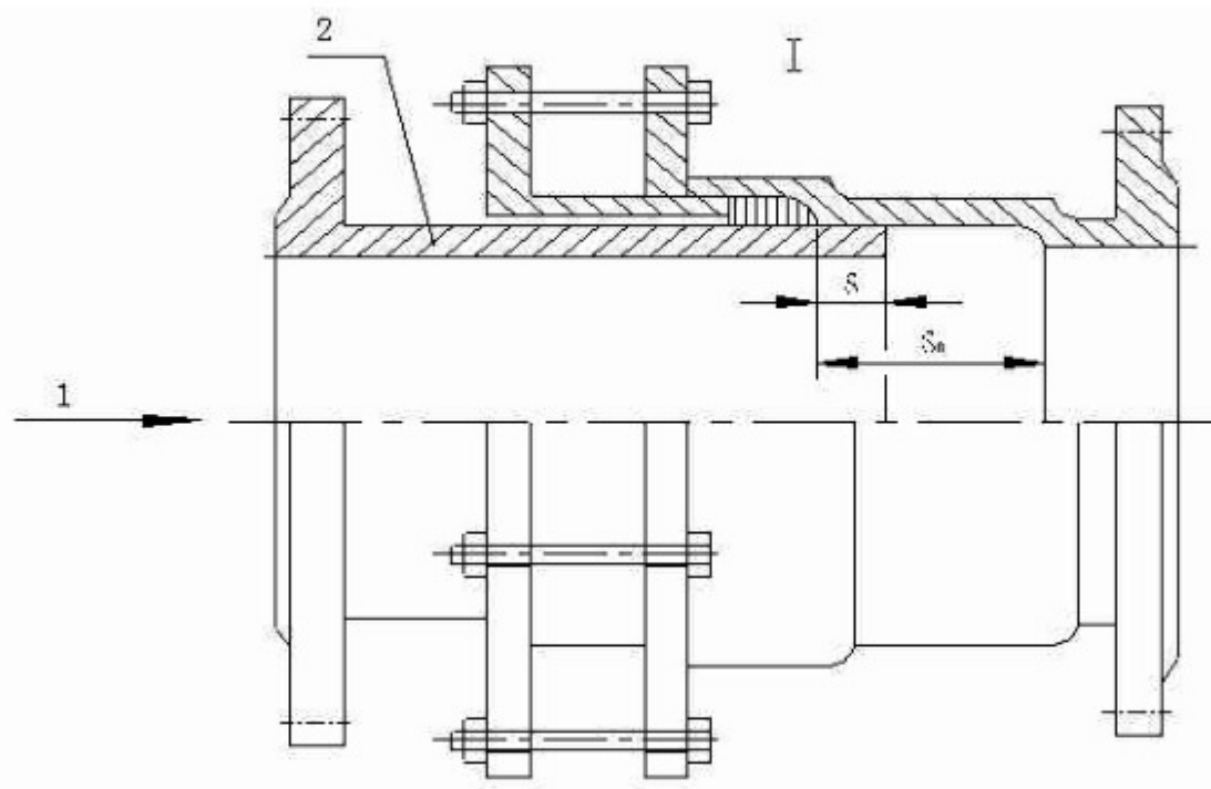
图 7.11.4 填料式补偿器安装剩余收缩量
