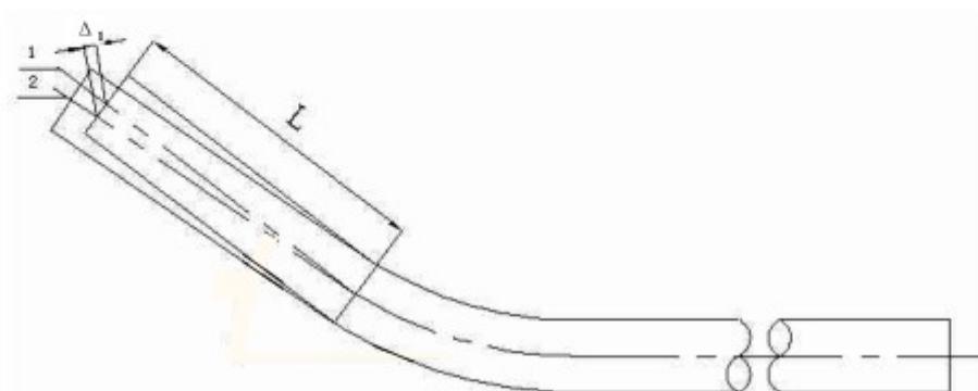
图 5.3.7-2 弯管的管端中心偏差
