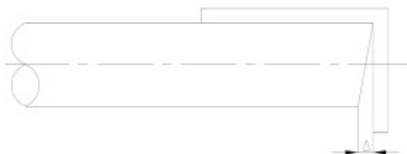
图 5.2.4 管子切口端面倾斜偏差
