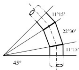
(c) 45° 斜接弯头
