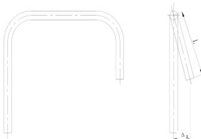
图 5.3.8 \Pi 形弯管平面度
