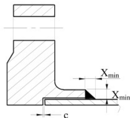
图 6.0.7-2 承插焊法兰与管子的连接
