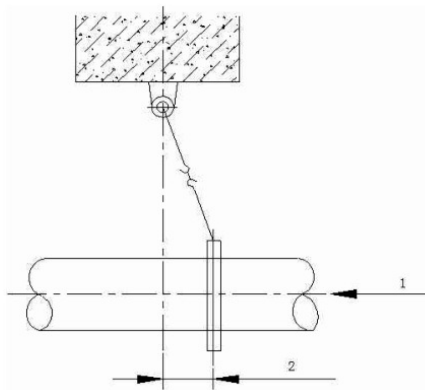
图 7.12.3 有热位移管道吊架安装
